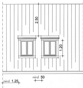
Rückwärtige Ansicht mit neuen Gauben
