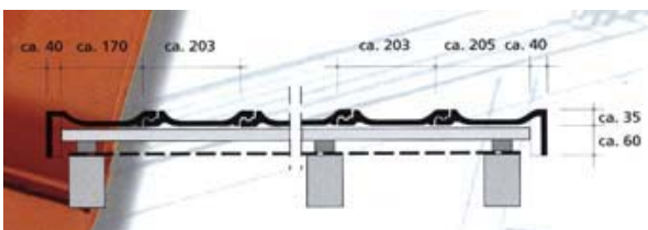
Ortgangziegel mit geringem Überstand
