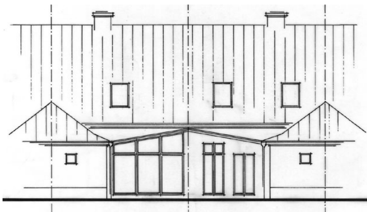
Höchster Punkt des Daches des neuen Anbaus unterhalb der Traufgesimse des Haupthauses
