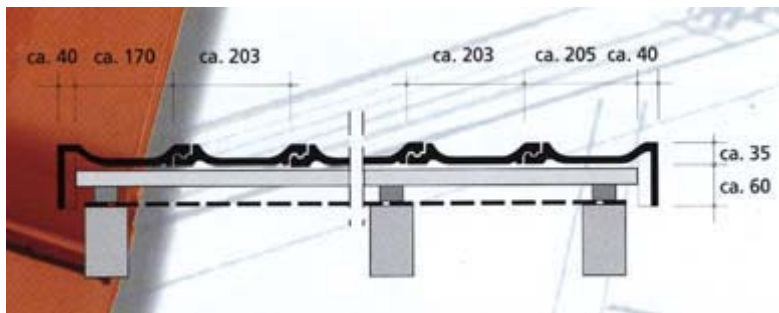
Ortgangziegel mit geringem Überstand
