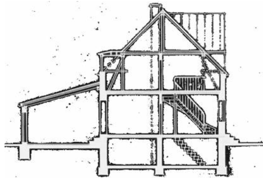
Schnitt mit neuem Anbau
