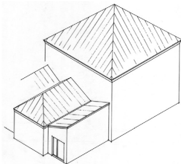
Versatz des Anbaus gegenüber dem Haupthaus
