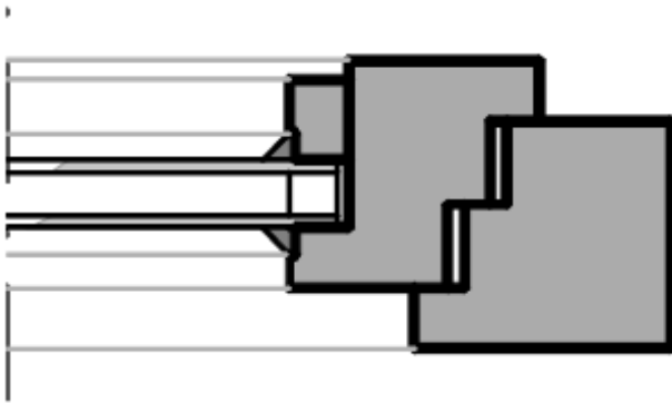
Horizontalschnitt: Flächenversetzte Profile
