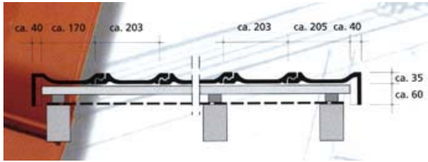
Ortgangziegel mit geringem Überstand
