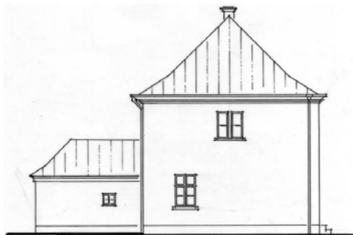
Seitenansicht mit historischem Anbau
