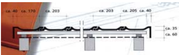
Ortgangziegel mit geringem Überstand
