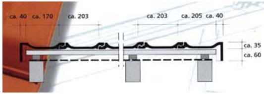
Ortgangziegel mit geringem Überstand
