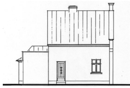
Seitenansicht mit historischem und neuem Anbau
