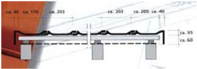
Ortgangziegel mit geringem Überstand
