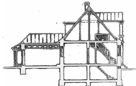
Schnitt mit altem und neuem Anbau
