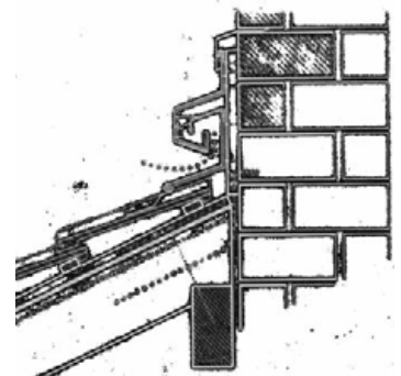
Beispiel für Dachanschluss Anbau /
