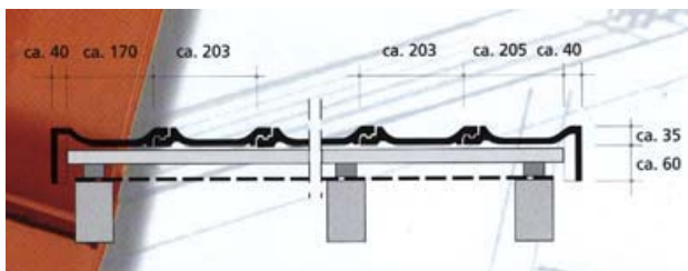
Ortgangziegel mit geringem Überstand
