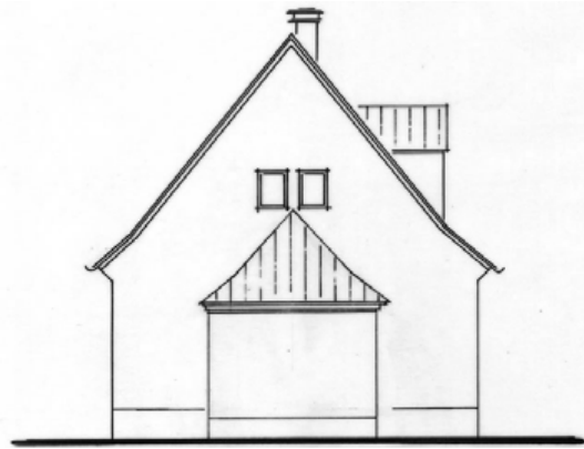
Seitenansicht mit seitlichem historischem Anbau
