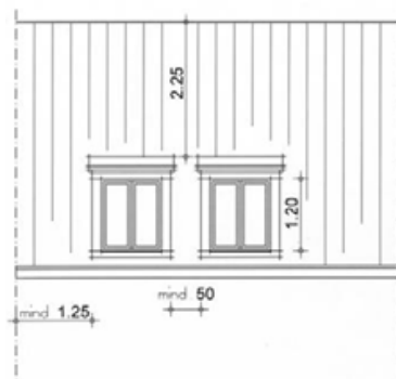
Rückwärtige Ansicht mit neuen Gauben
