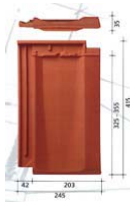
Tondachziegel vom Typ Rheinland
