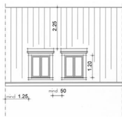
Rückwärtige Ansicht mit neuen Gauben
