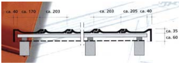
Ortgangziegel mit geringem Überstand
