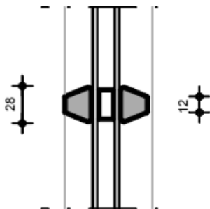
Vertikalschnitt: Aufgesetzt Sprossen
