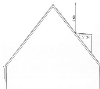
Seitenansicht mit neuer Gaube
