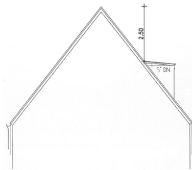
Seitenansicht mit neuen Gauben
