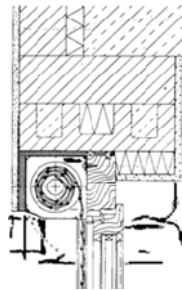
Vertikalschnitt: Rollladenanschluss mit Fertigsturz
