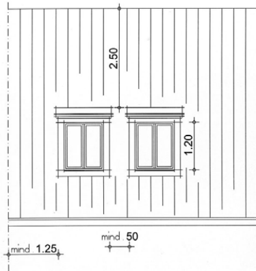
Rückwärtige Ansicht mit neuen Gauben
