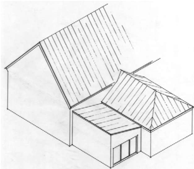
Versatz des Anbaus gegenüber dem Haupthaus bei rückwärtigem historischem Anbau
