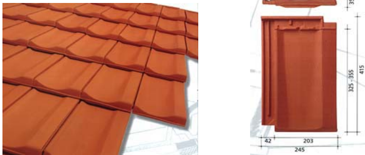
Tondachziegel vom Typ Rheinland
