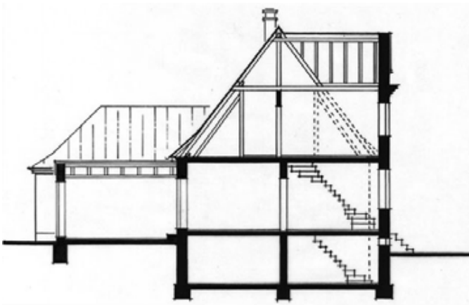
Schnitt des historischen Gebäudes mit altem und neuem Anbau
