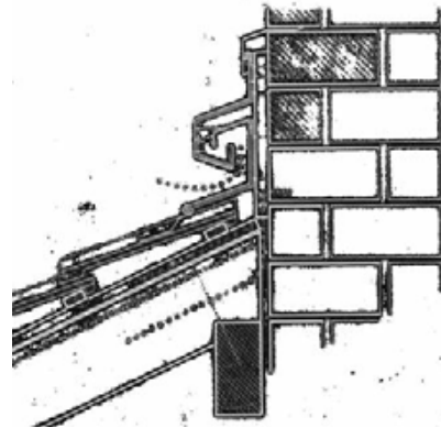
Beispiel für Dachanschluss Anbau / Haupthaus
