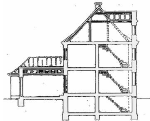
Schnitt des historischen Gebäudes mit altem und neuem Anbau
