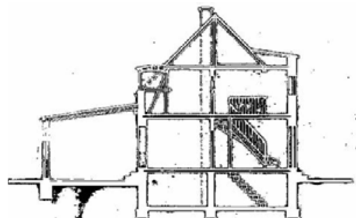
Schnitt mit neuem Anbau
