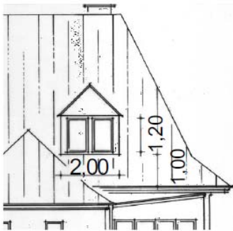
Rückwärtige Ansicht mit neuer Gaube
