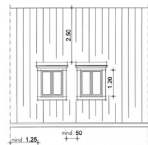
Rückwärtige Ansicht mit neuen Gauben
