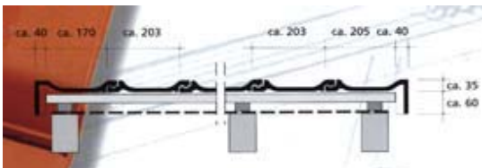
Ortgangziegel mit geringem Überstand
